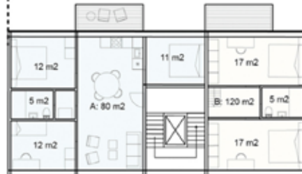
2. etage
